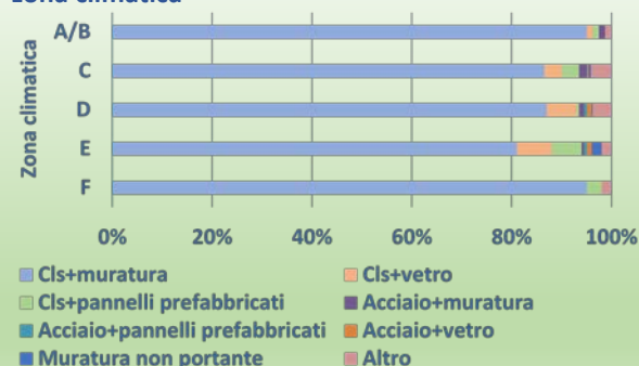
Figura 5.1 - Edifici scolastici: tipologie costruttive per zona climatica
