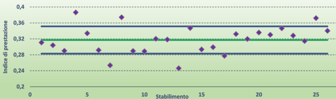
Figura 4.6 – Indice di prestazione generale di stabilimento per la produzione di tissue
