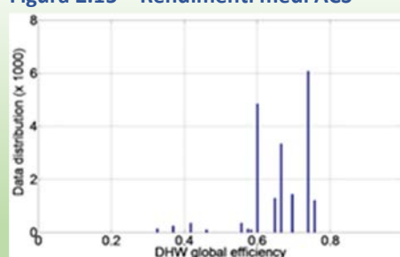
Figura 2.15 – Rendimenti medi ACS
