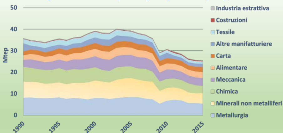
Figura 2.10 – Consumo energetico nell'industria per comparto produttivo (Mtep), anni 1990-2015
