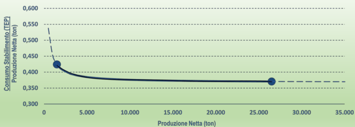
Figura 4.5 – Indice di prestazione energetica generale per lo stabilimento di una fonderia di ghisa
