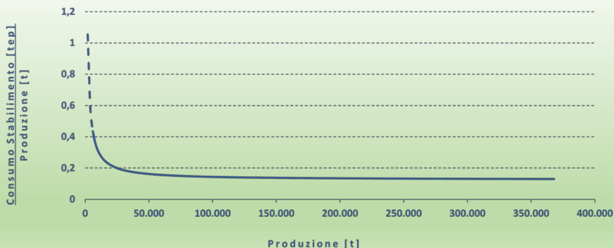
Figura 4.7 – Indice di prestazione generale di stabilimento per la produzione di ceramica
